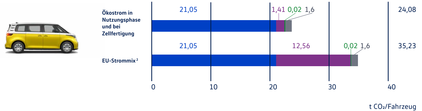
Vollständige CO 2 -Emissionen nach Lebenszyklusphase: ID. Buzz 150 kW 82 kWh (brutto) (Modelljahr 2024) 1
