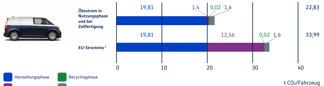
Vollständige CO 2 -Emissionen nach Lebenszyklusphase: ID. Buzz Cargo 150 kW 82 kWh (brutto) (Modelljahr 2024) 1
